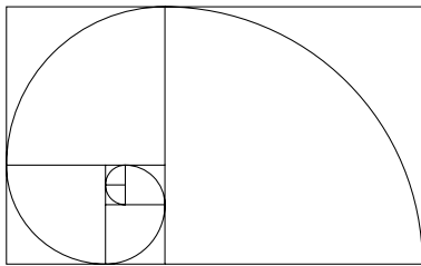
Figura 4 – Representação gráfica da sequência de Fibonacci.
